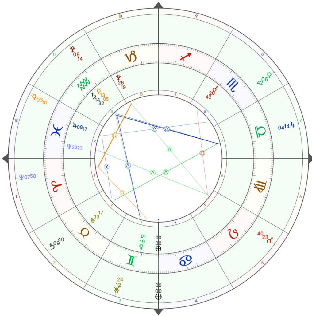
Carta heliocéntrica, Rueda interior: inicio 6.1, Solsticio de diciembre del 2021. Rueda exterior: inicio 7.1, Solsticio de diciembre del 2027.
