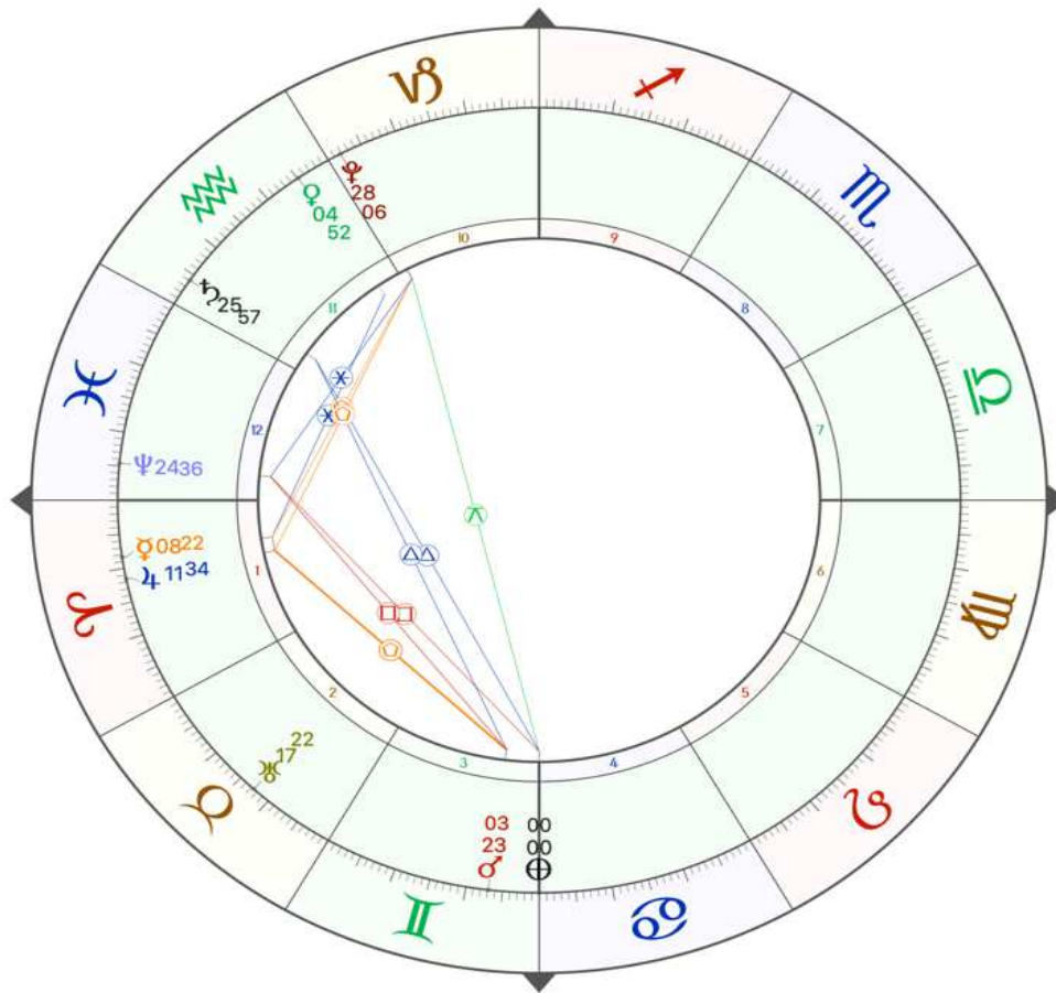
Solsticio, 21 de diciembre del 2022; 22:48 horas, CET.
