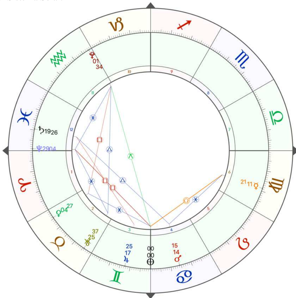
Solsticio, 21 diciembre del 2024; 10:20 horas, CET.
