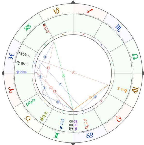
Solsticio 21.12.2024, 10:22 horas; Inicio del Año 6.4 / 2025
