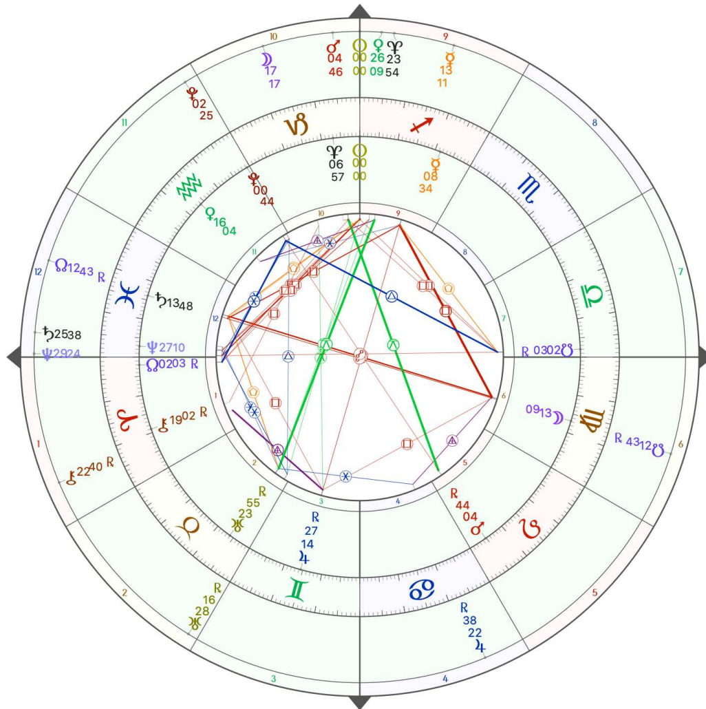
Rueda interior: Solsticio 21.12.2024, 10:22 h. - Rueda exterior: Solsticio 21.12.2025, 16:04 h.
